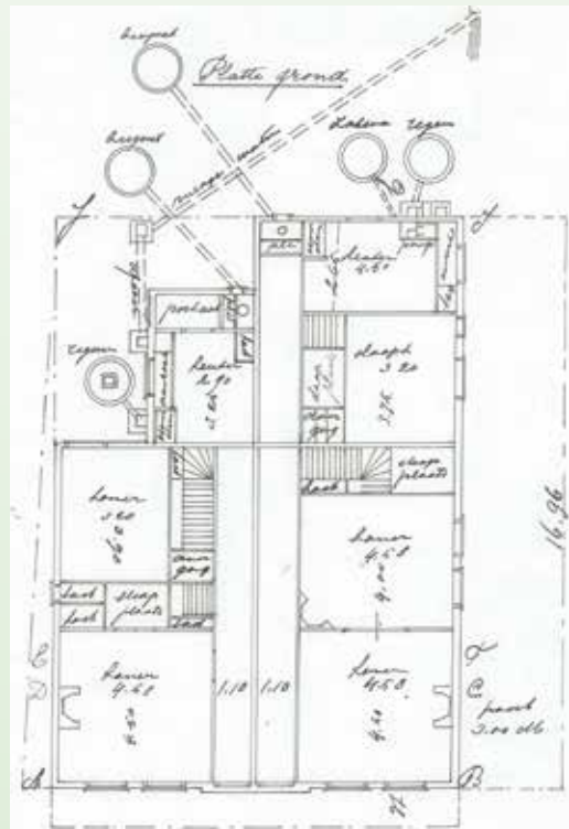
De plattegrond en de zolder met de kamers (gespiegeld) van het nieuwe kosthuis, 1909 (Stadsarchief Zoetermeer)
