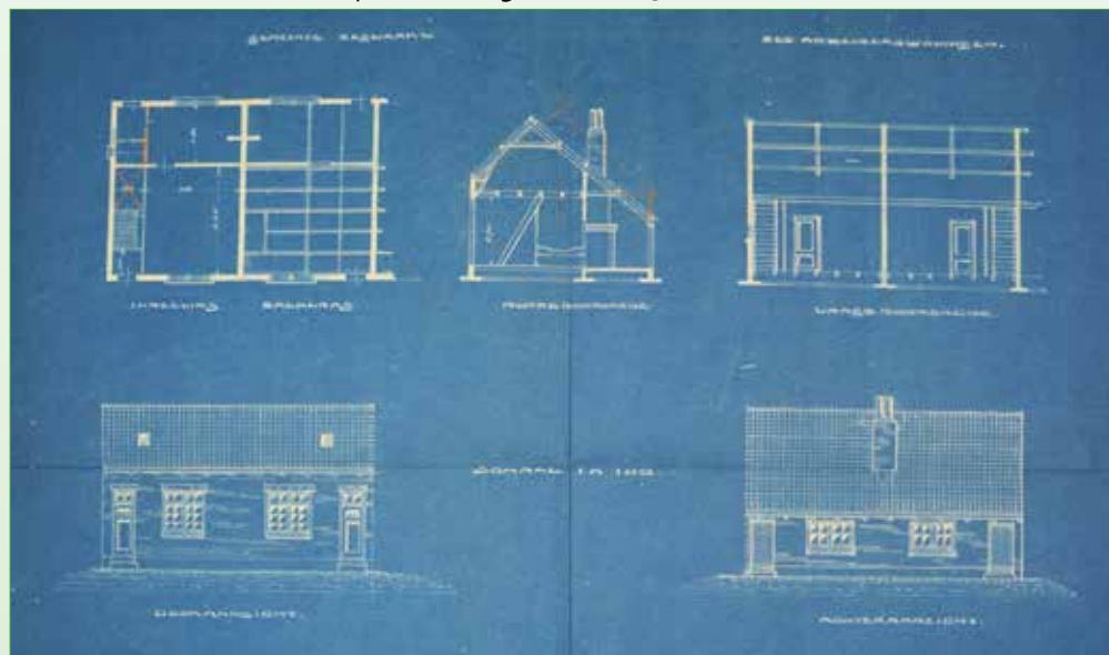
Het eerste bouwplan voor noodwoningen, 1922 (Nationaal Archief, Hoofdinspectie Volksgezondheid 906)
