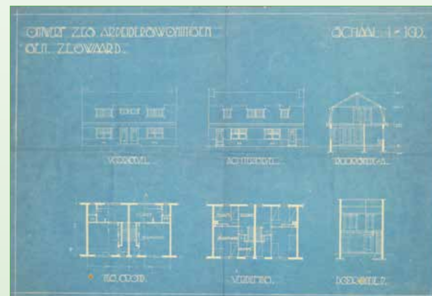
Bouwtekening voor de uiteindelijk gerealiseerde woningen (Stadsarchief Zoetermeer, Gemeentebestuur Zegwaart 1092)
