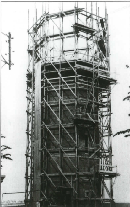
De bouw van de Watertoren bij de Stationsstraat is halverwege, 1927. (Collectie Oud Soetermeer)
