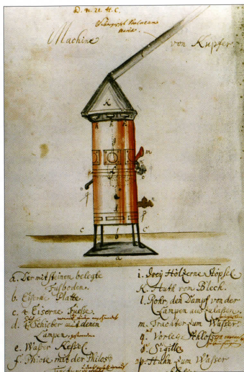
De ketel uit het stookhuis van Syberg te Memmingen. De afbeelding bevindt zich in de processtukken aldaar. (Stadtarchiv Memmingen A 168/01; A 168/02; A 169/01; A 170/01). Met dank aan Peter Altena.
