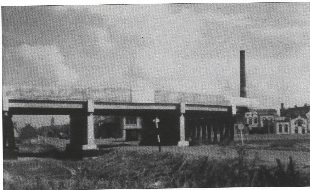
Voor de aanleg van de rijksweg waren kunstwerken nodig, waaronder het viaduct over de Stationsstraat in Zoetermeer, dat in 1930 werd gebouwd ( W. van Gool, Voorburg)
