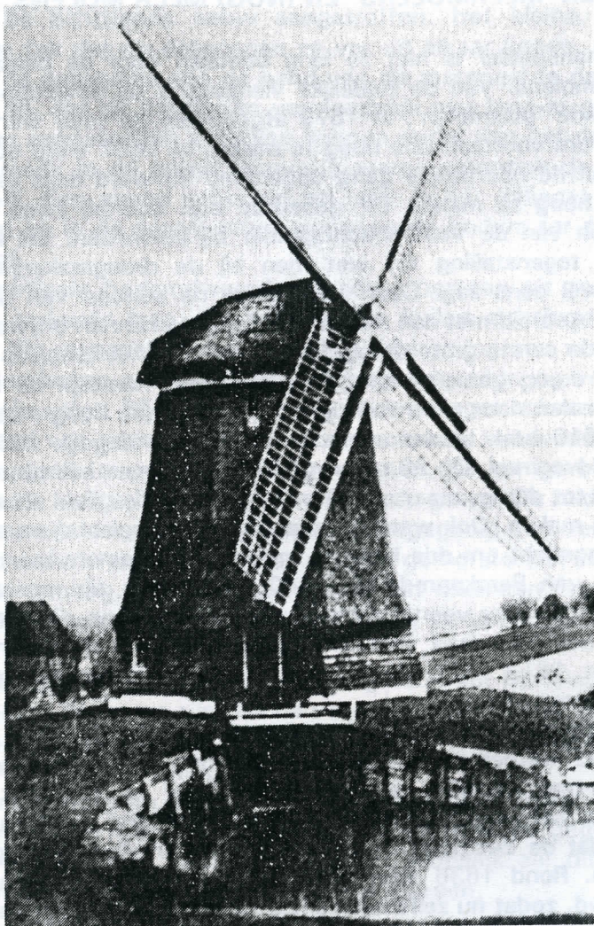
De bovenste middelmolen van de Rijpergang in De Beemster (gesloopt in 1885). De molen was een zgn. 'binnenkruier', d.w.z. het op de wind zetten, het kruien, van kap met wieken gebeurde binnen, boven in de molen.
