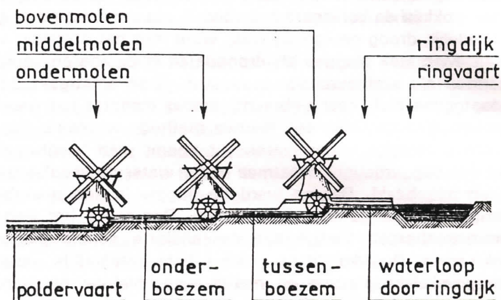
Getrapte bemaling door een gang van drie molens.
